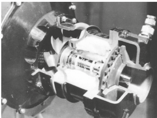
Turbochladičí jednotka. | Foto: Archiv PBS
