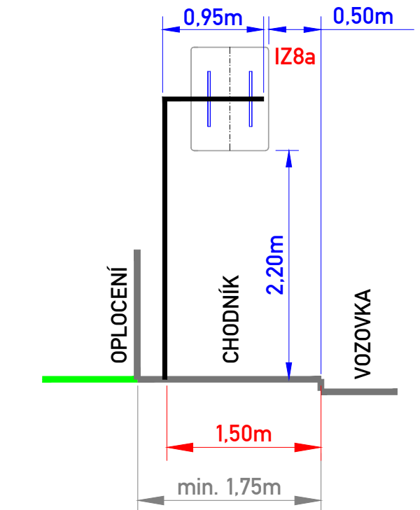
VZOROVÉ OSAZENÍ SVISLÉHO DZ
