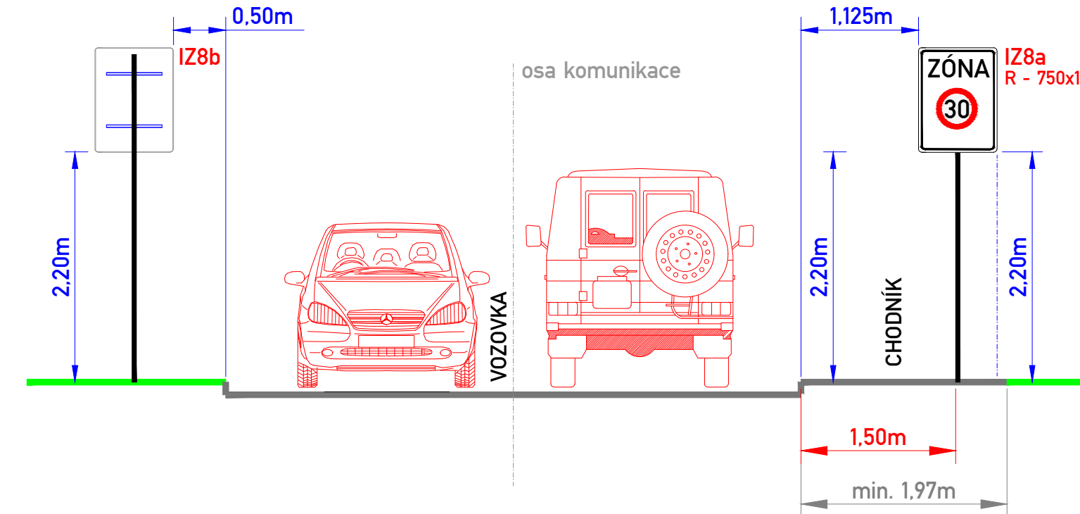
ŘEZ B-B OSAZENÍ SVISLÉHO DZ
